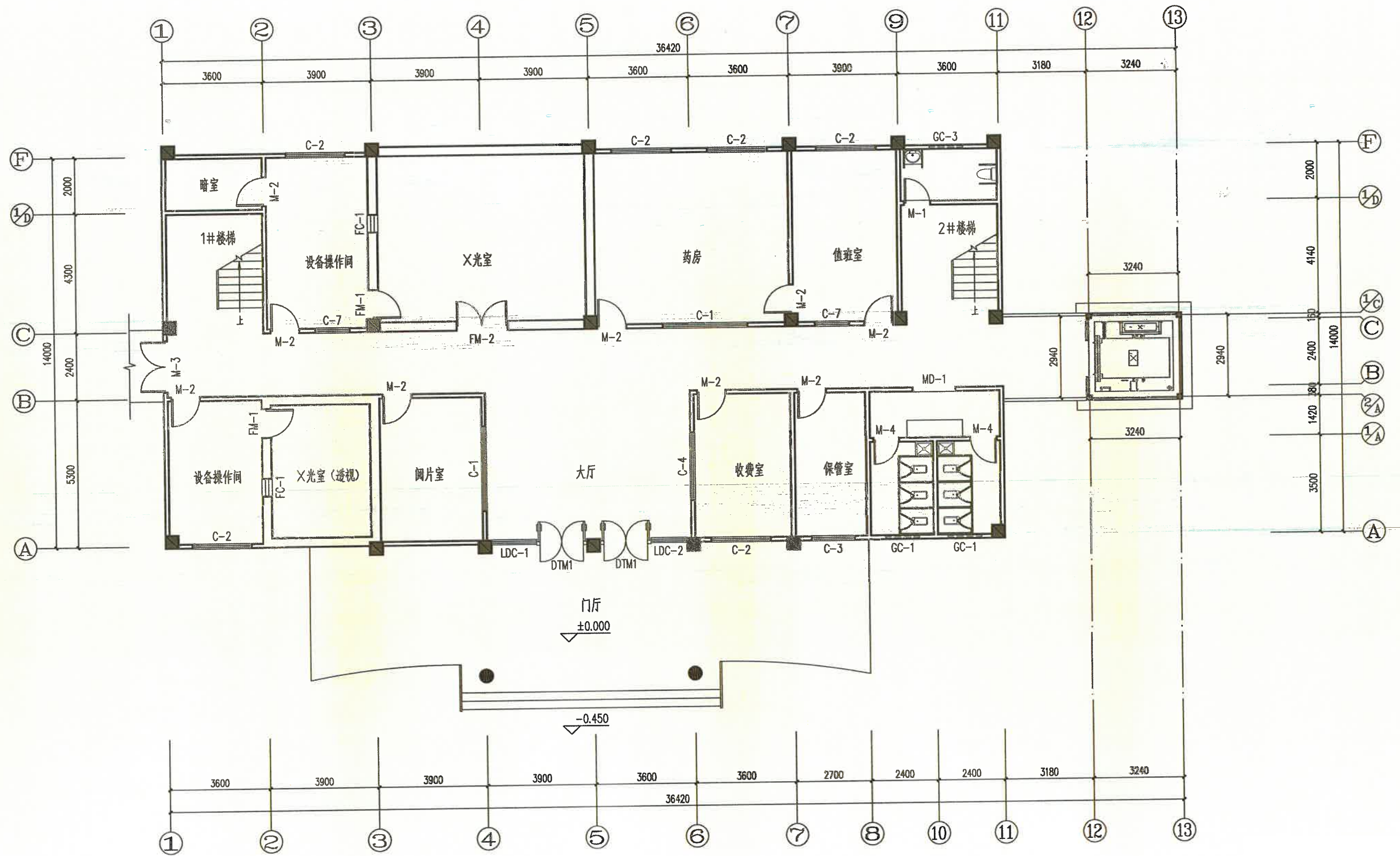
一层平面图 1:100
